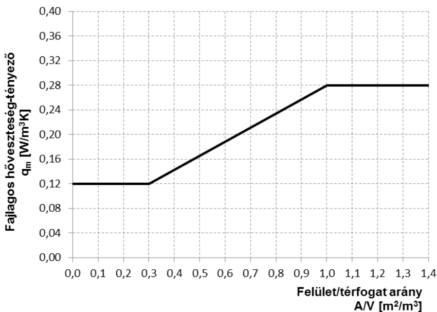
1. ábra: A fajlagos hővesztesség-tényező követelményértéke.
